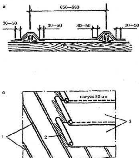
Рис. 5. Покрытие стальных кровель рулонными материалами: а — рядами параллельно коньку; б — рядами перпендикулярно коньку; 1 — прижимные гребнистые чих фальцев; 2 — горячий битум; 3 — рубероид
